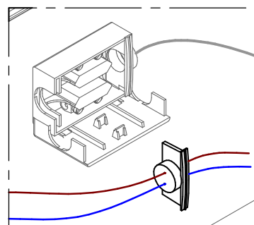
DETTAGLIO A
